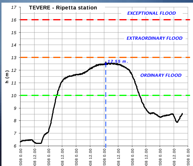
Soglie di Frosini (1977) per Ripetta
