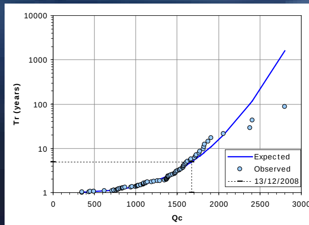
Ripetta (distribuzione normale)
