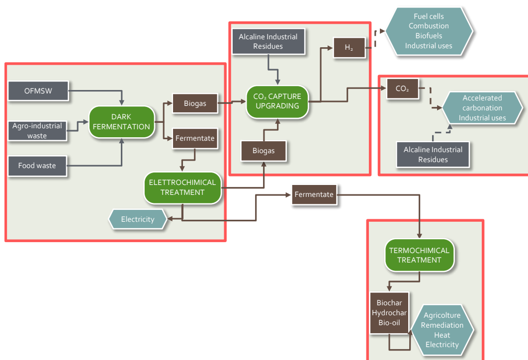
LAYOUT DEL PROCESSO BBcIRLE
