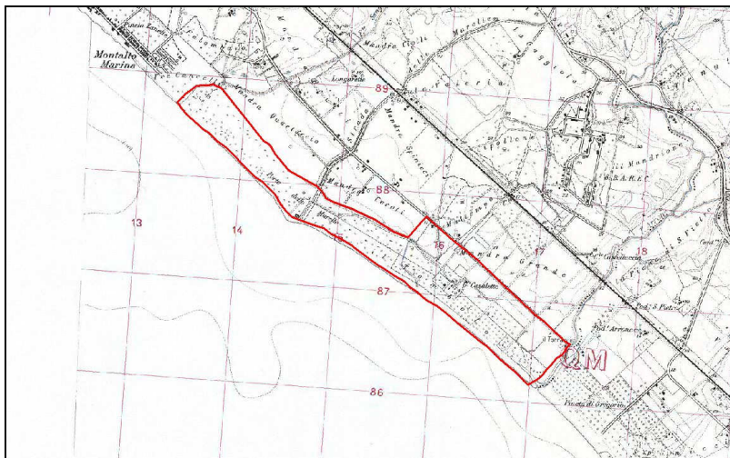
Cartografia del SIC "Litorale tra Tarquinia e Montalto di Castro"
